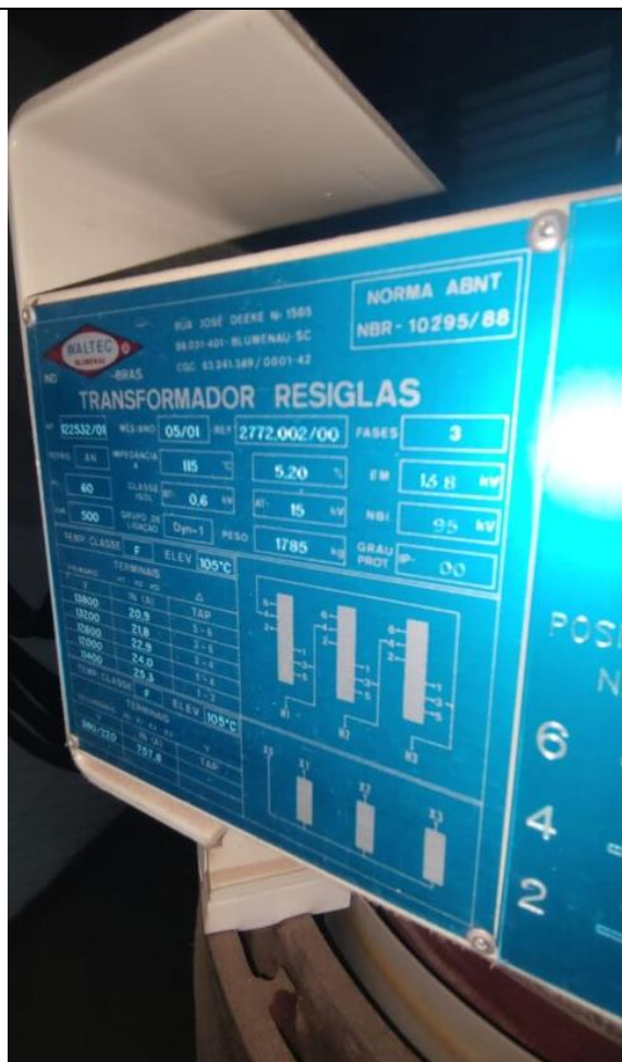
1. Trafo 500kVA a seco
